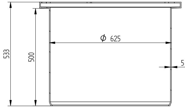
SECTION D-D
